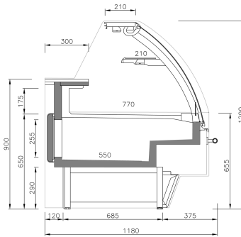
VBC RU/RIU (con reserva) [Whit storage] [Avec réserve]
