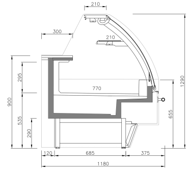
VBC SU/SIU (Sin reserva) [Whitout storage] [Sans réserve]
